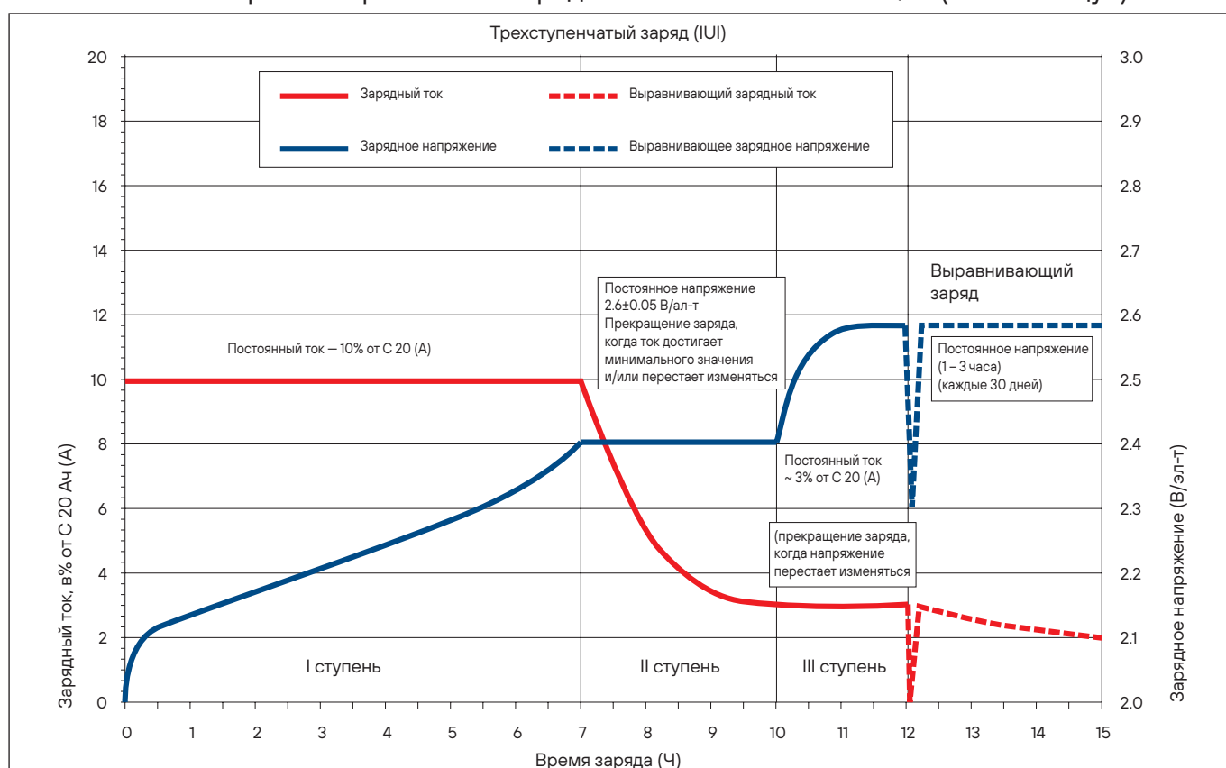
Схема 2. Рекомендуемый график заряда аккумуляторных батарей с жидким электролитом IUI.
