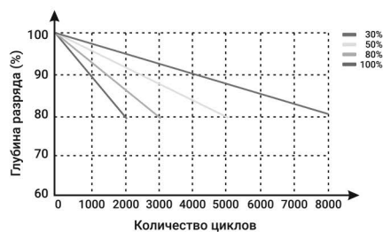
Ресурс/Глубина разряда (DOD)
