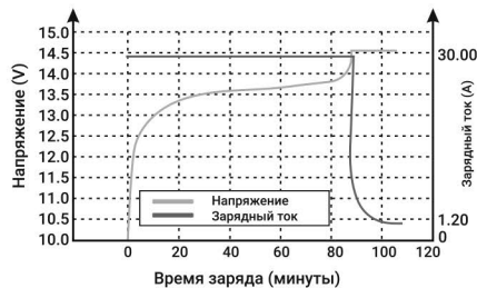
Зарядные характеристики(0.5C)
