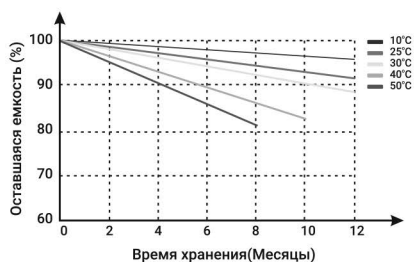
Саморазряд/Температура
