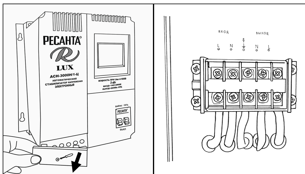
Рис. 6. Клеммная колодка
