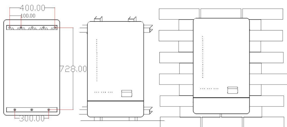
Настенный монтаж
