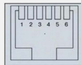
Интерфейс обмена данными RS232
