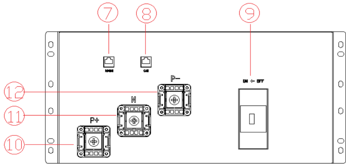
Батарейный модуль
