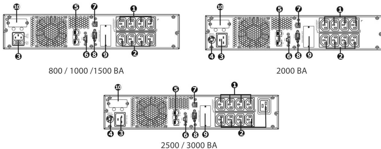
Рис 1-1 Вид сзади
