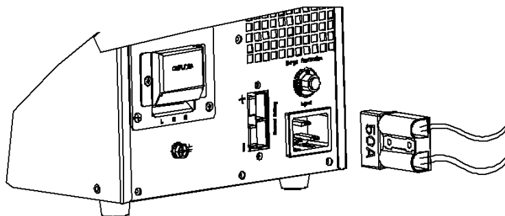
Рисунок 5. Подключение батареи
