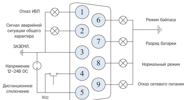
Порт DB9 (9-контактный разъём)
