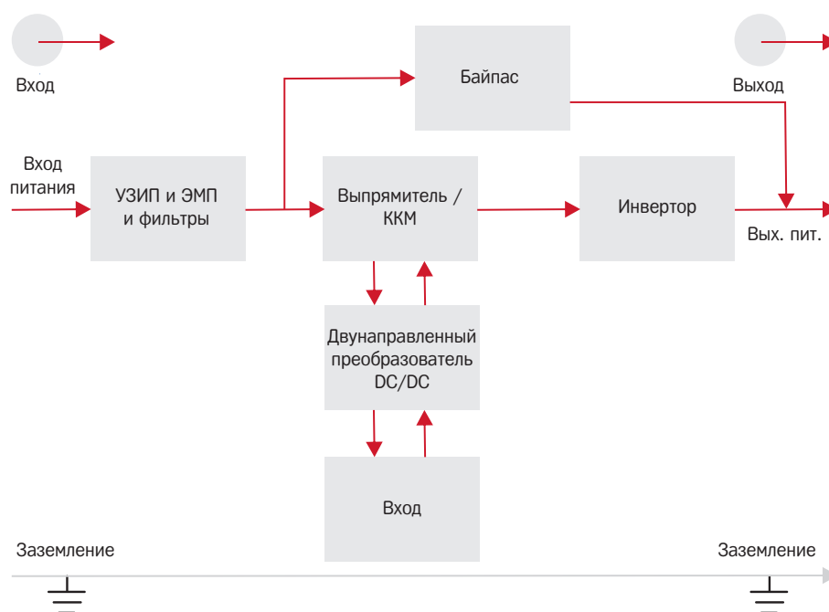
Рисунок 3. Схема системы
