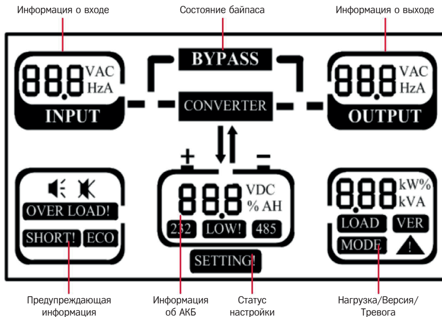
Рисунок 7. Меню ЖК-дисплея
