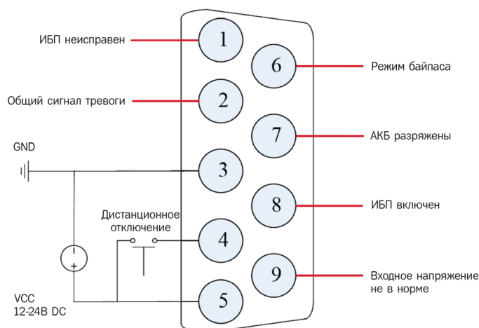
Рис. 9-1 Схема подключения сухих контактов
