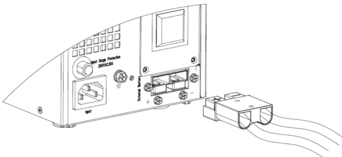
Рис. 4-2 Подключение АКБ
