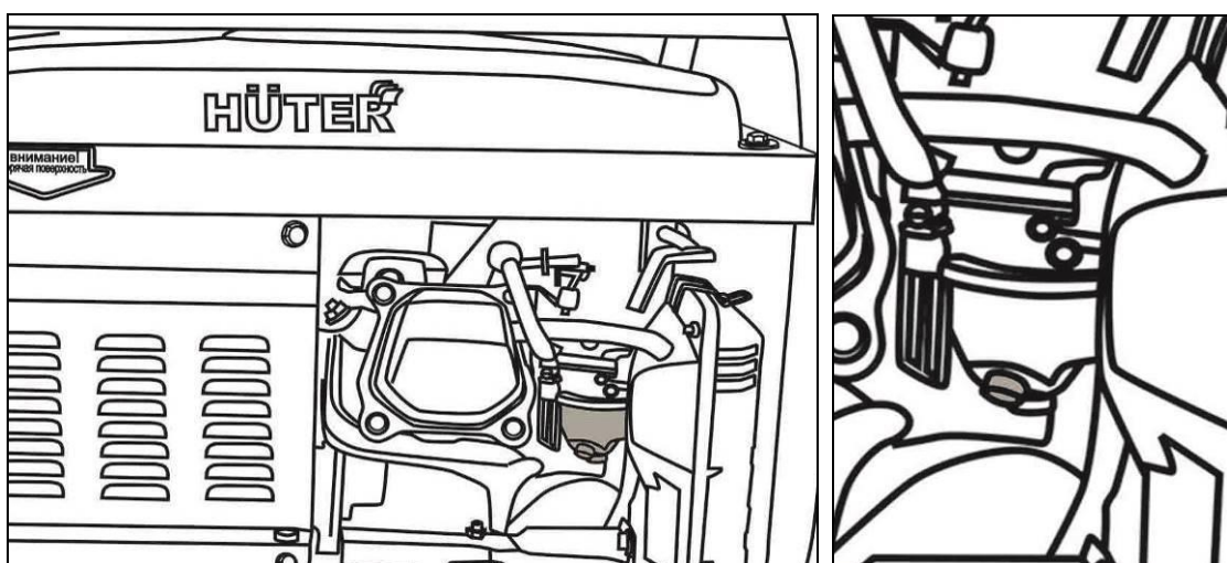
Рис. 18. Слив топлива из карбюратора
