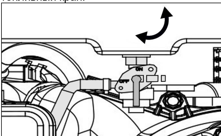
Рис. 8. Топливный кран
