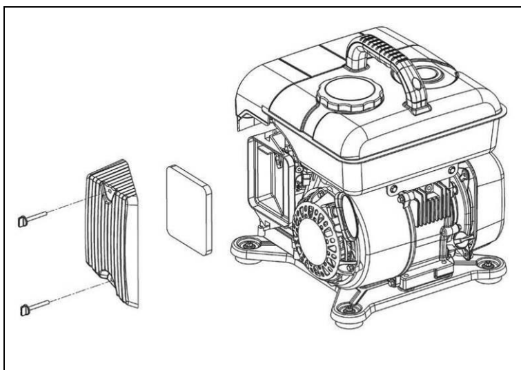
Рис. 16. Воздушный фильтр
