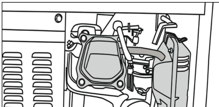
Рис. 12. Трубка сапуна.
