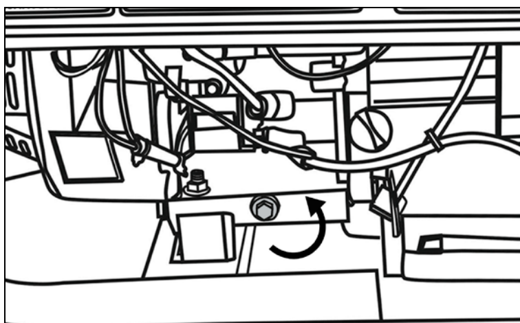
Рис. 13. Слив масла
