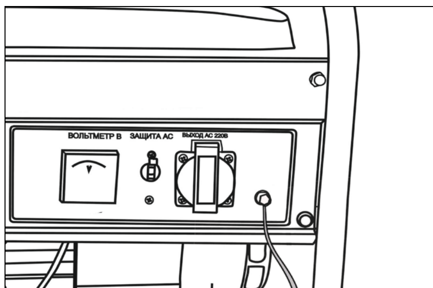
Рис. 4. Заземление
