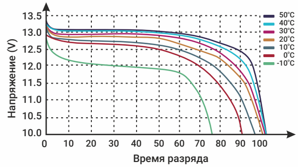
Температура/Время разряда
