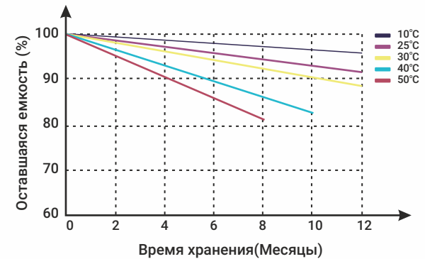
Саморазряд/Температура
