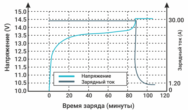
Зарядные характеристики
