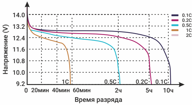
Напряжение/Время разряда
